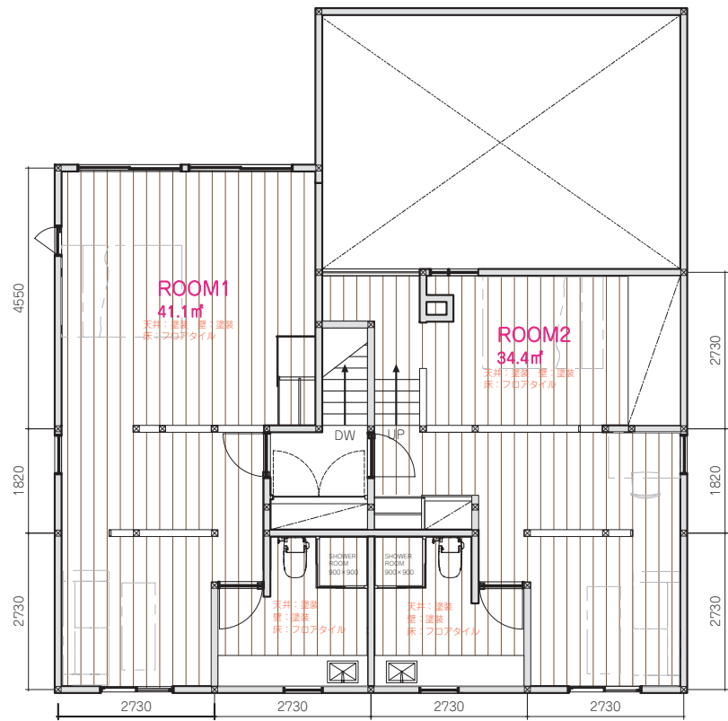
◎2F 平面図 S=50:1
