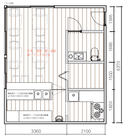
◎別棟 平面図 S=50:1
